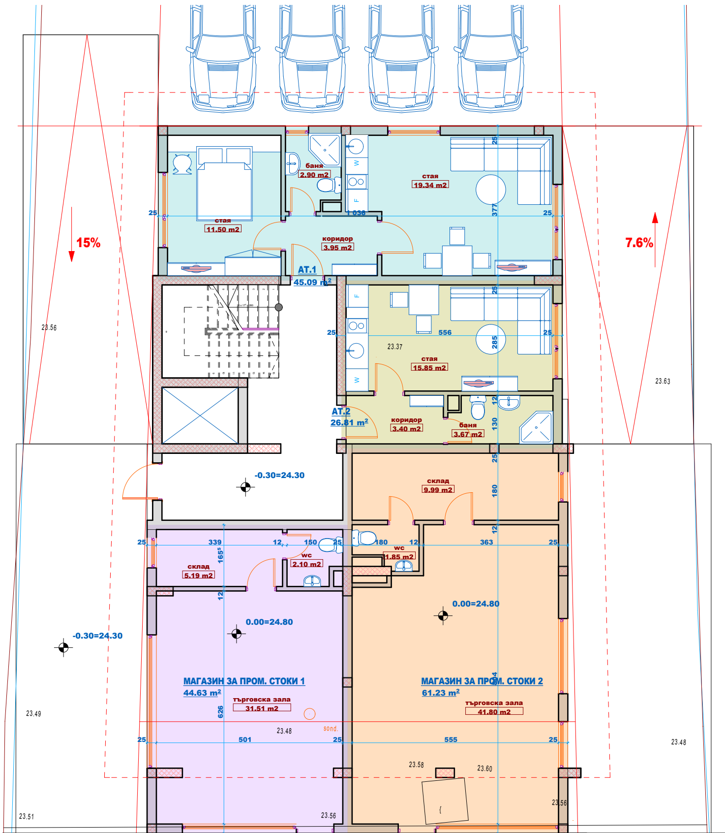
СГРАДА 1 РАЗПРЕДЕЛЕНИЕ ПАРТЕР застроена площ 211кв.м.
