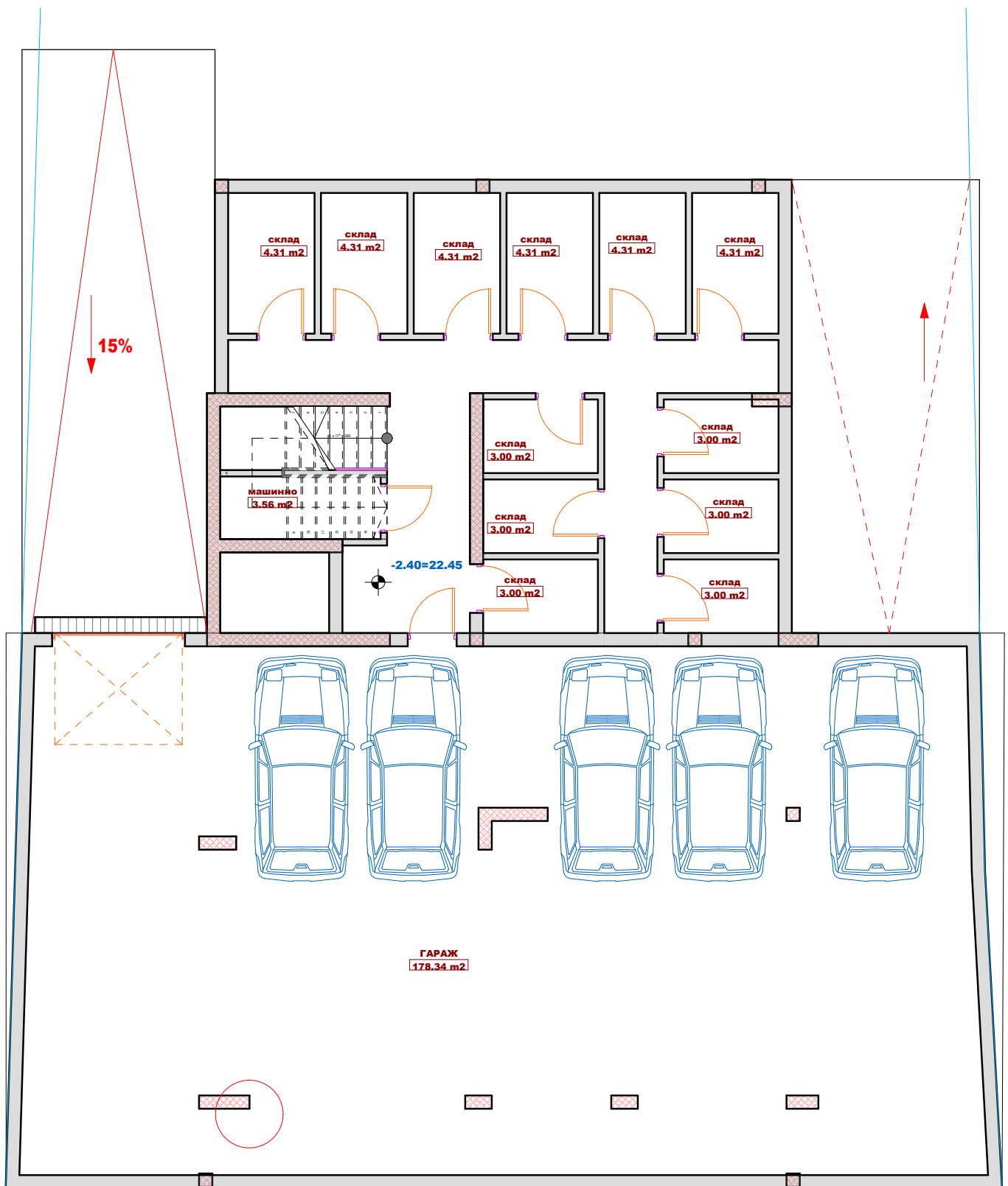
СГРАДА 1 РАЗПРЕДЕЛЕНИЕ СУТЕРЕН застроена площ 285.50кв.м.
